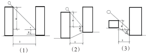
图1 南北方向2栋建筑的关系
